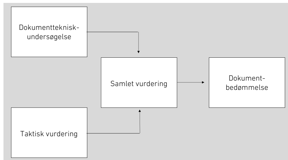
Figur 2: Todelt dokumentbedømmelsesmetode.
