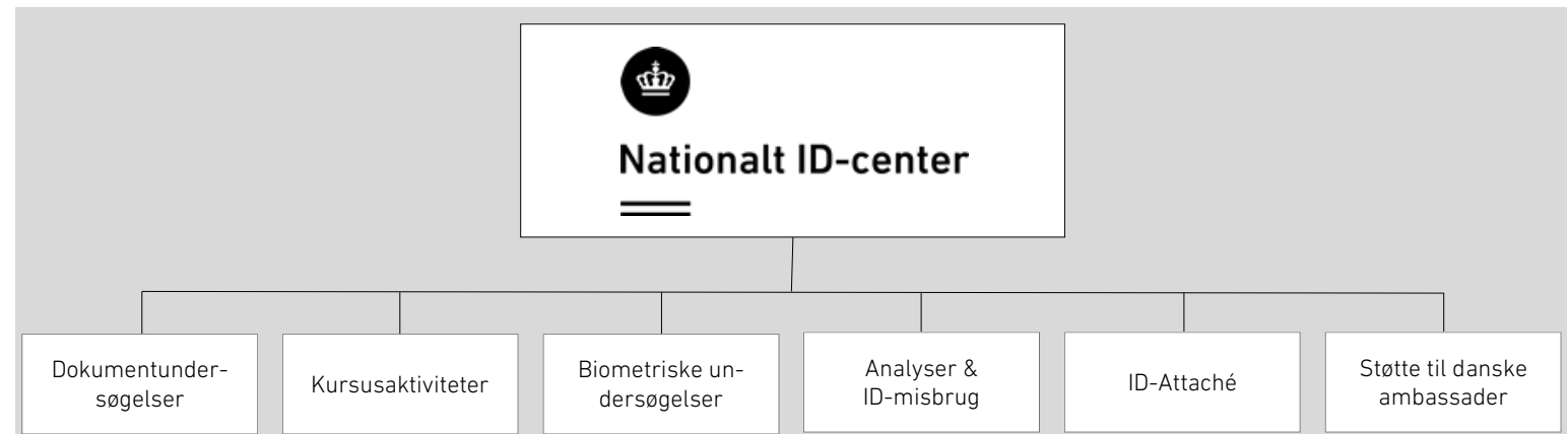
Figur 1: NIDC opgavediagram.
